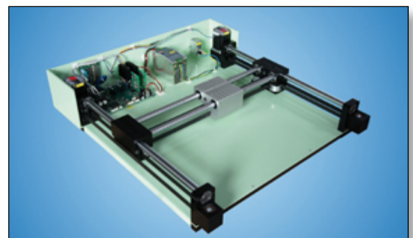
DriveSet M227E mit integrierter Steuerung (Abdeckung geöffnet)
